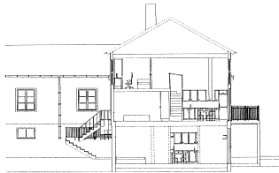
Sektion B 1:100
