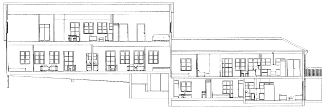
Sektion A 1:100
