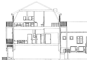
Sektion C 1:100
